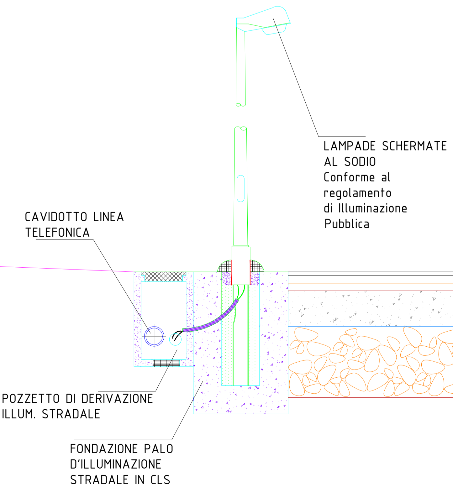
PARTICOLARE POZZETTO
