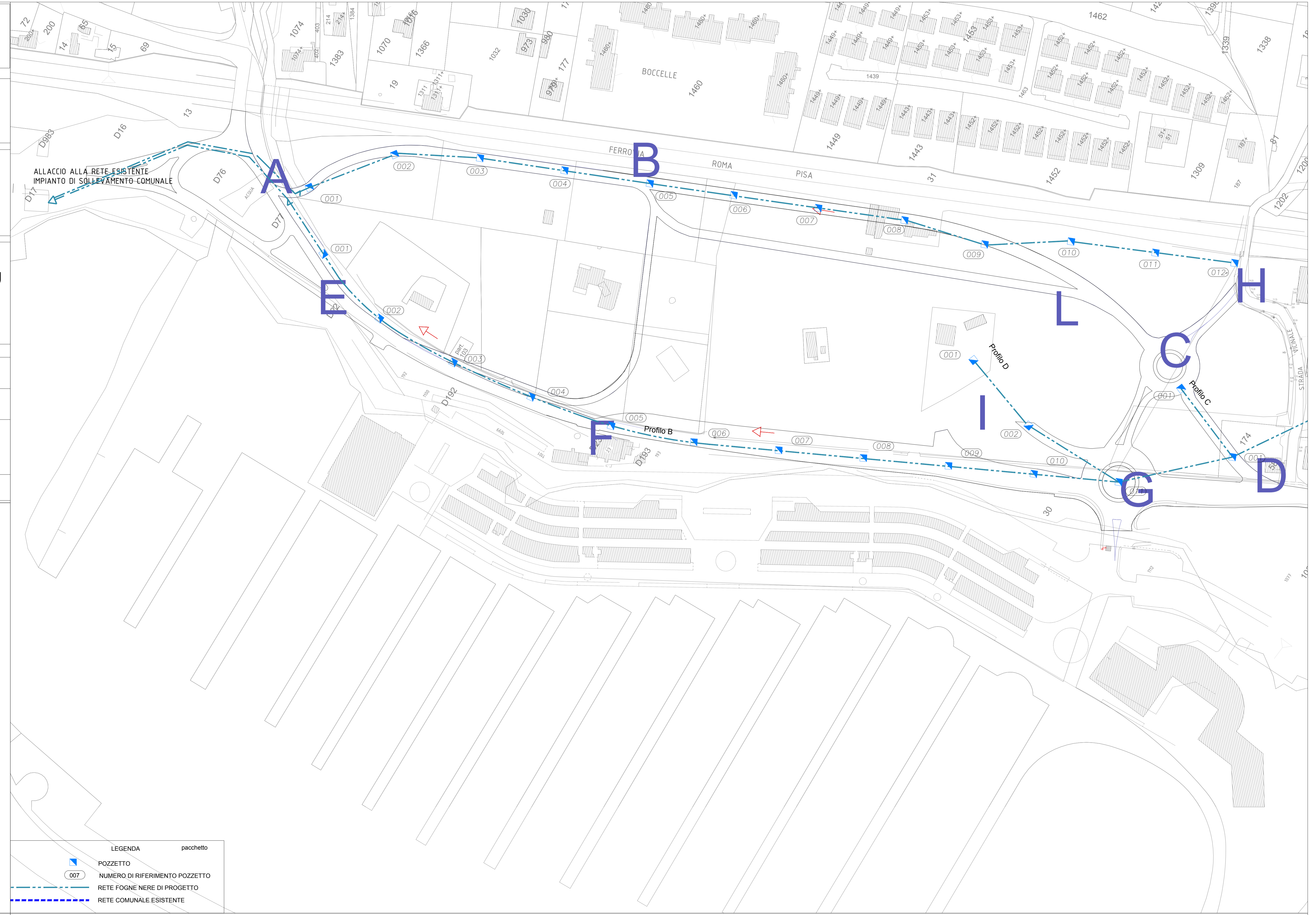
PLANIMETRIA scala 1: 1000
