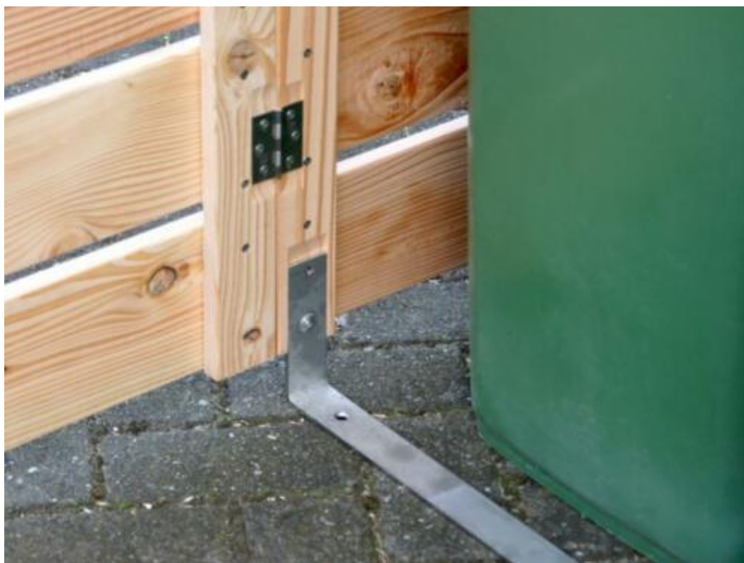
Illustrazione 6: esempio di aggancio al suolo
