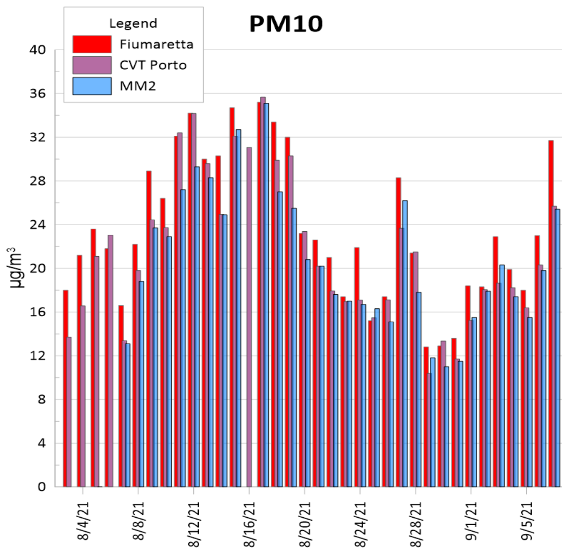
Figura 2: Valori giornalieri di PM10 nel periodo suddetto per il MM2, Civ. Porto e Fiumaretta
