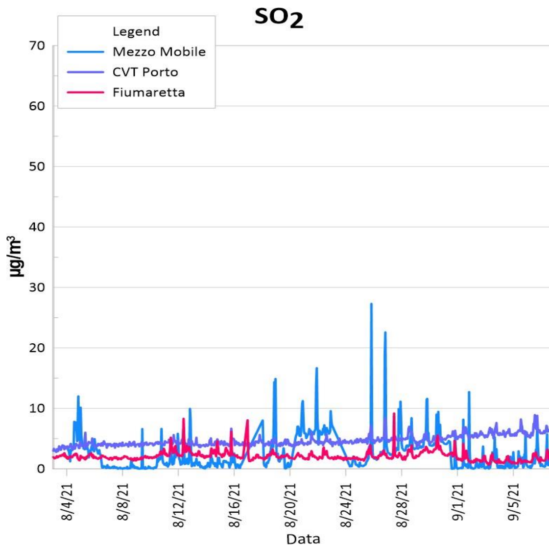
Figura 8: Valori orari di SO 2 nel periodo suddetto per il MM2, Civ. Porto e Fiumaretta
