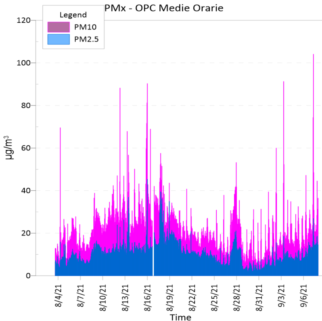
Figura 4: Valori di PM10 e PM2.5 nel periodo suddetto misurati ogni 15 minuti
