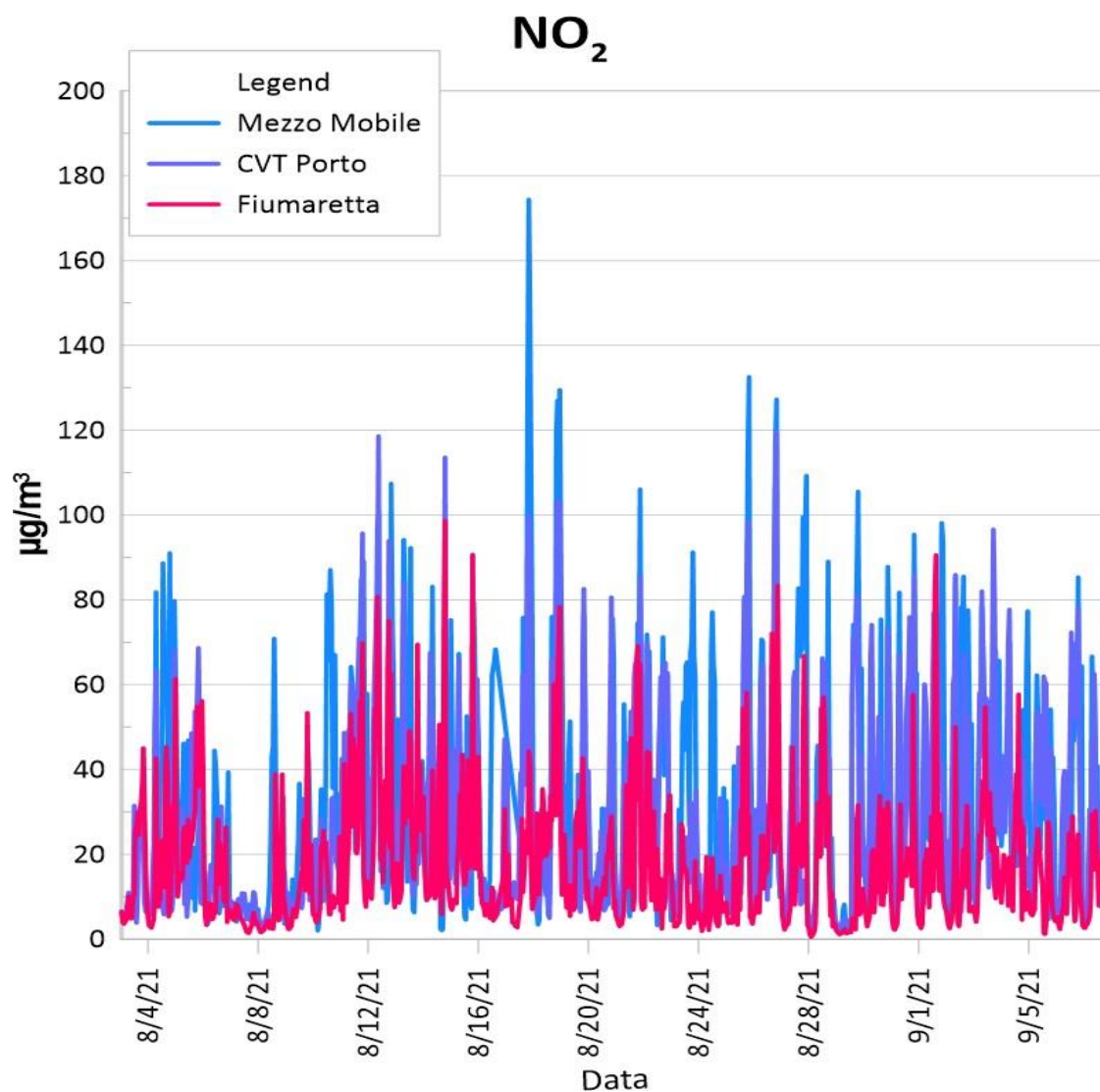
Figura 5: Valori orari di NO 2 nel periodo suddetto per il MM2, Civ. Porto e Fiumaretta
