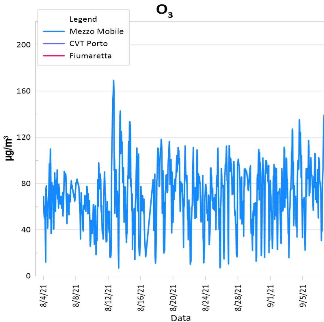
Figura 7: Valori orari di O 3 nel periodo suddetto per il MM2
