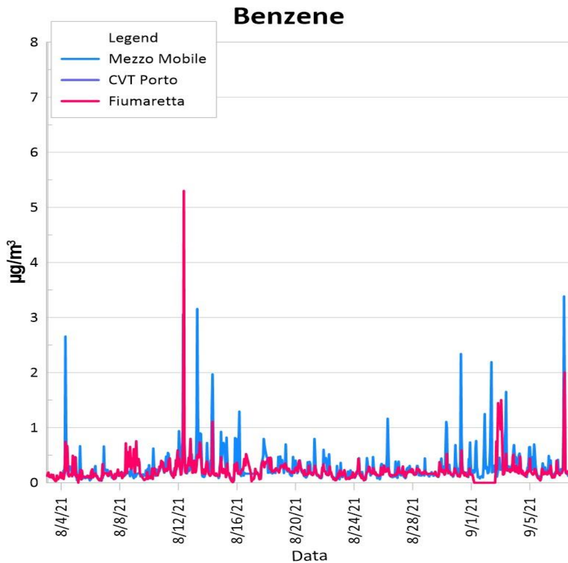
Figura 9: Valori orari di Benzene nel periodo suddetto per il MM2 e Fiumaretta
