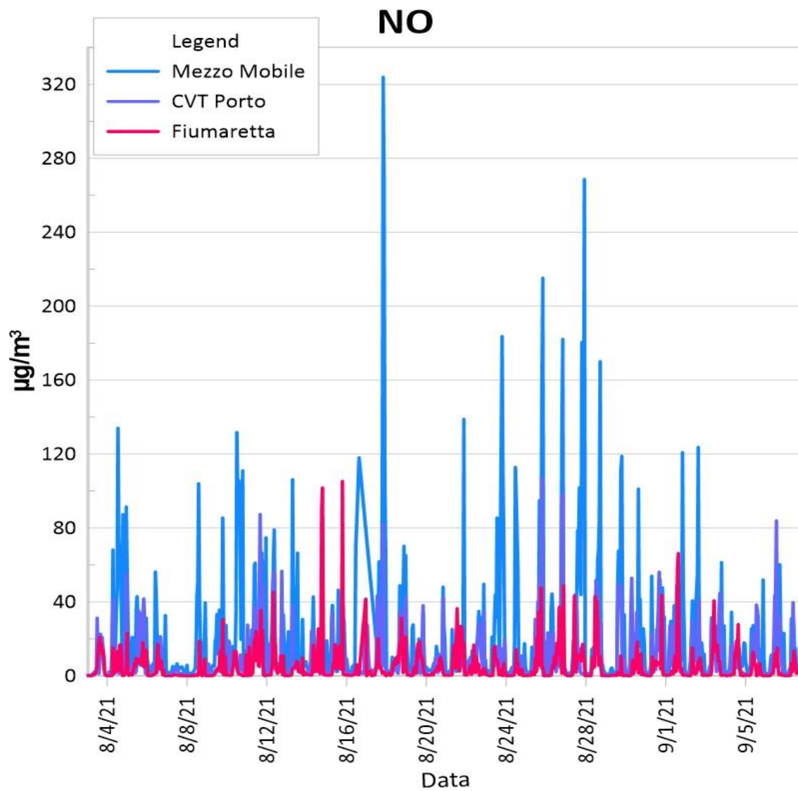
Figura 6: Valori orari di NO nel periodo suddetto per il MM2, Civ. Porto e Fiumaretta
