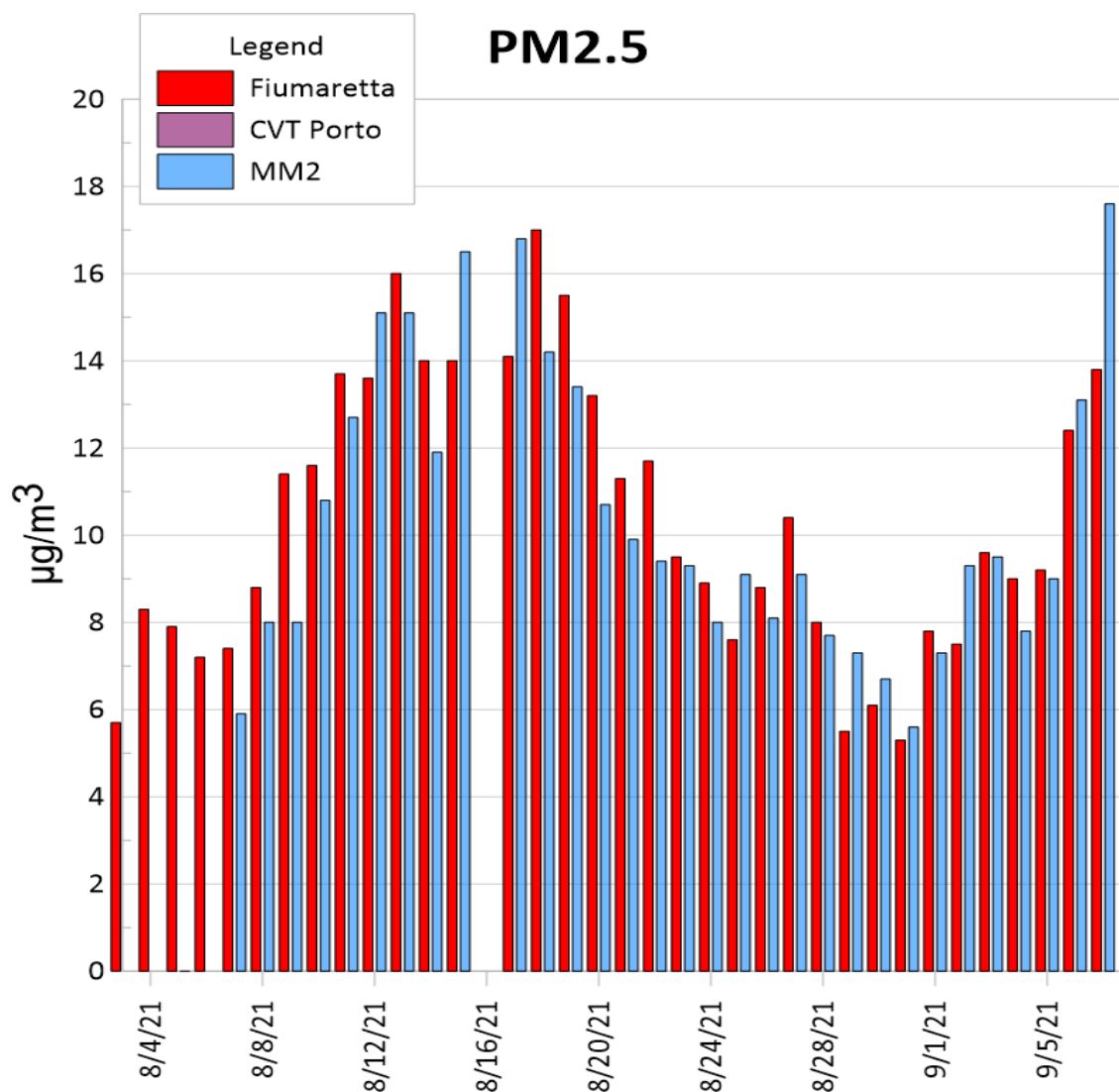
Figura 3: Valori giornalieri di PM2.5 nel periodo suddetto per il MM2 e Fiumaretta
