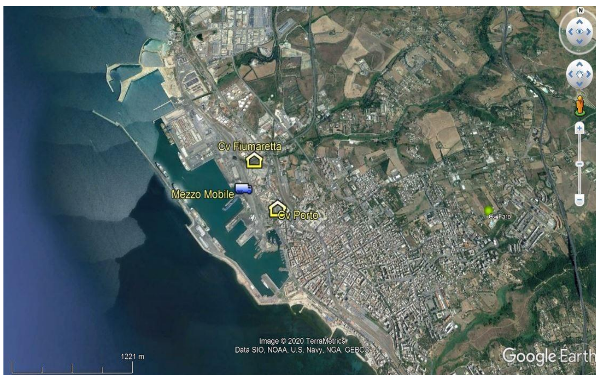
Figura 1: Mezzo Mobile presso il Porto di Civitavecchia e stazioni di misura fisse di Fiumaretta e Civitavecchia Porto distanti dal Mezzo Mobile circa 400 e 500 metri rispettivamente.
