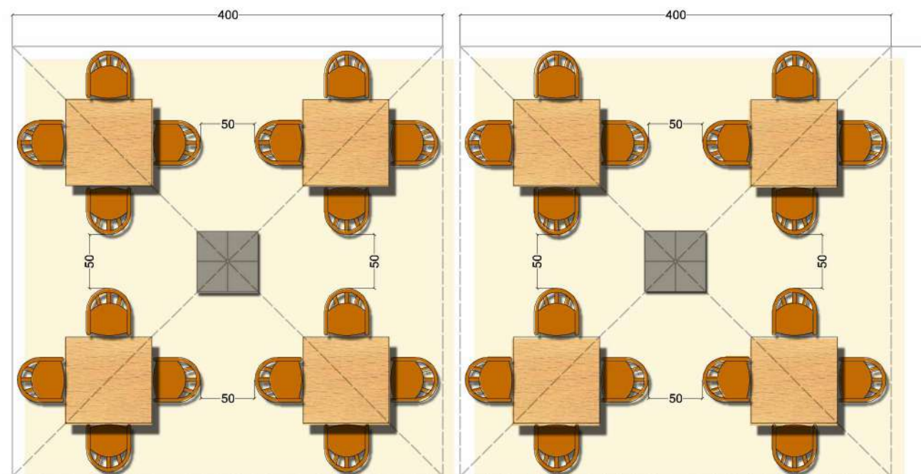
IPOTESI DI SISTEMAZIONE PLANIMETRICA UTILIZZANDO DUE OMBRELLONI DI M. 4,00 X 4,00, RICAVANDO N.32 POSTI A SEDERE
