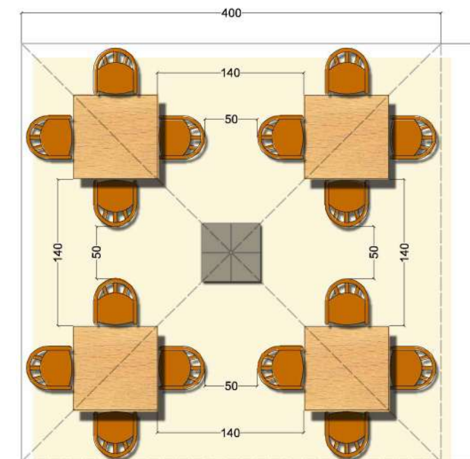
ESEMPLIFICAZIONE DI POSIZIONAMENTO DI TAVOLI E SEDIE ENTRO UN'AREA DI M 4,00 X4,00 (DIMENSIONI DI OMBRELLONE TIPO)
