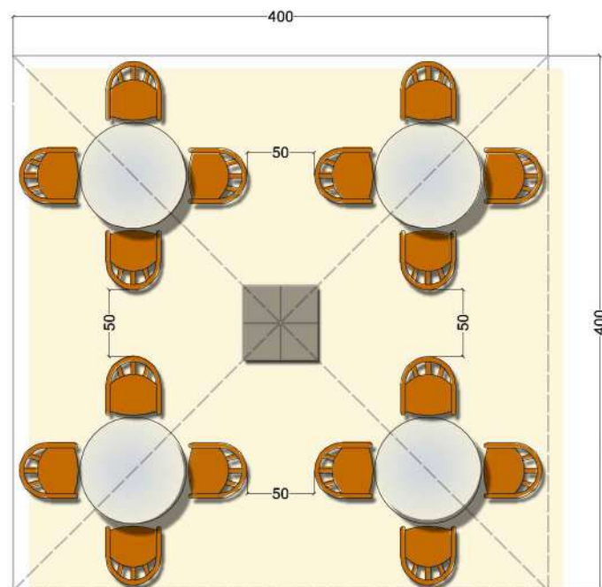
ESEMPLIFICAZIONE DI POSIZIONAMENTO DI TAVOLI E SEDIE ENTRO UN'AREA DI M 4,00 X4,00 (DIMENSIONI DI OMBRELLONE TIPO)
